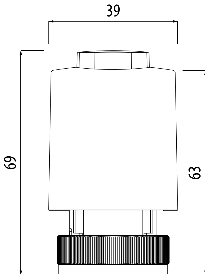
Rysunek wymiarowy
