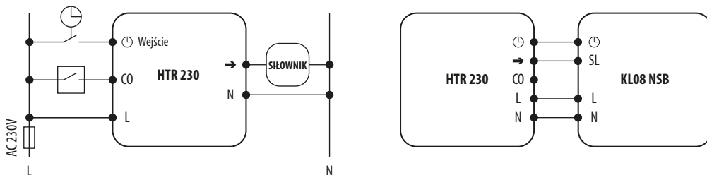
Schemat podłączenia
